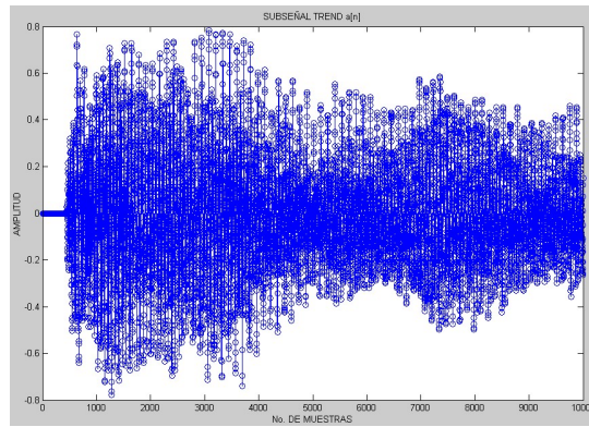
Fig. 6. Gráfica de la subseñal promedio a[n] de la transformada wavelet Haar
