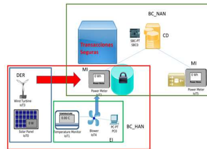
Fig. 3. Almacenamiento de datos general de la arquitectura de cadena de bloques propuesta
