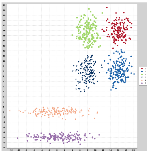
Fig. 2. Dataset longsquare
