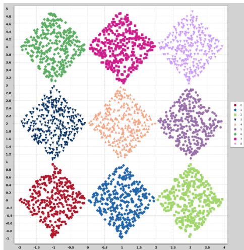
Fig. 1. Dataset diamond9
